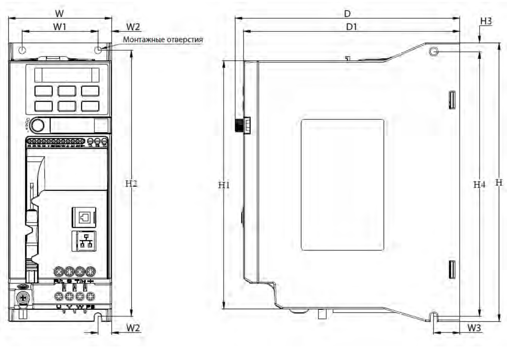
Рис.2-6.2. Чертеж преобразователя частоты типоразмер A2
