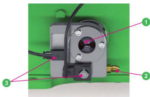
Регулятор уровня масла OLM-IQ
