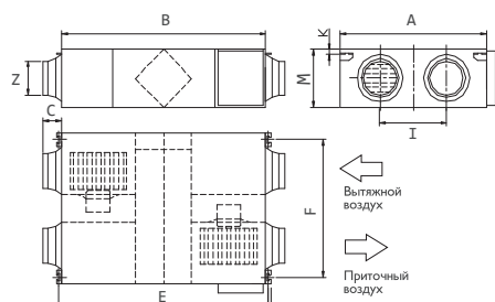
Модель RCS-250-P
