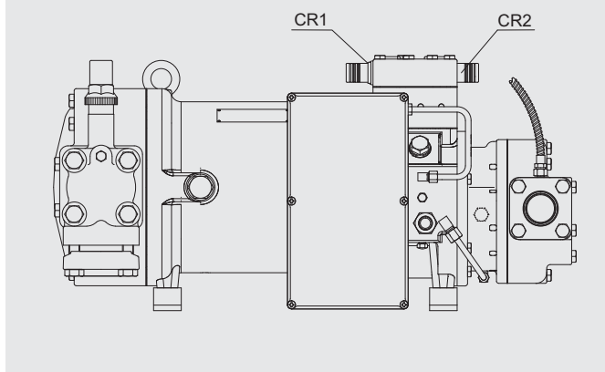
Abb. 5 Anordnung der Magnetventile
