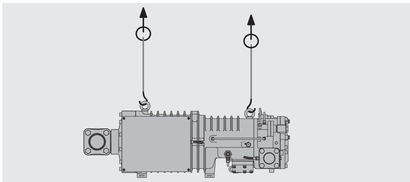
Abb. 1 Verdichter anheben
