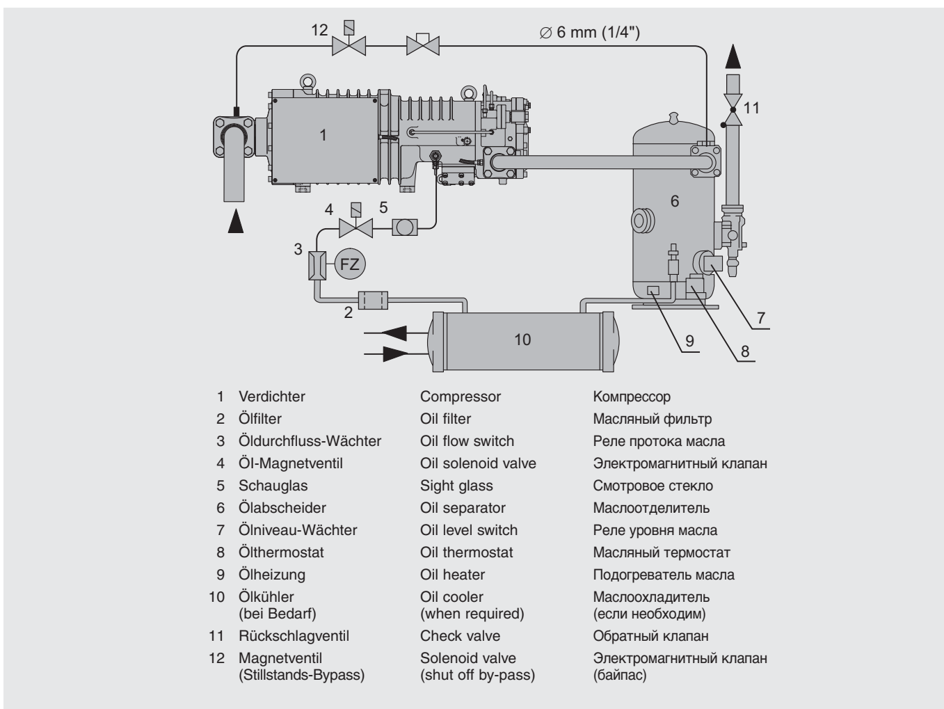
Abb. 6 Schmierölkreislauf
