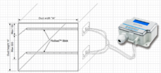
Рис. 2. Монтаж FloXact™-L
